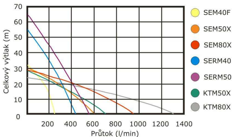
Závislost výtlaku na průtoku
